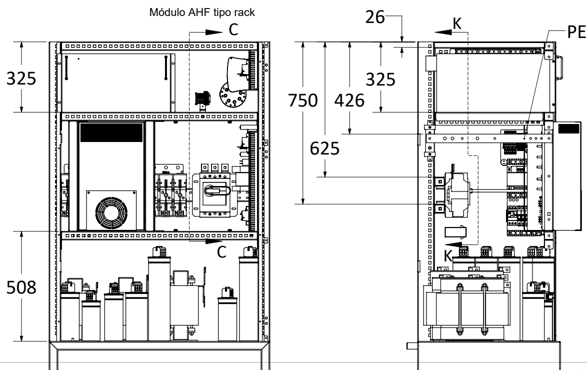
Módulo AHF tipo rack
